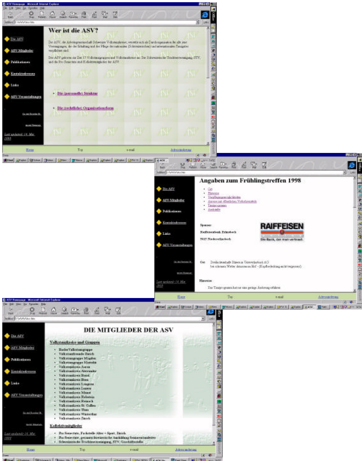
Abb. 1: Die ASV-Homepage
